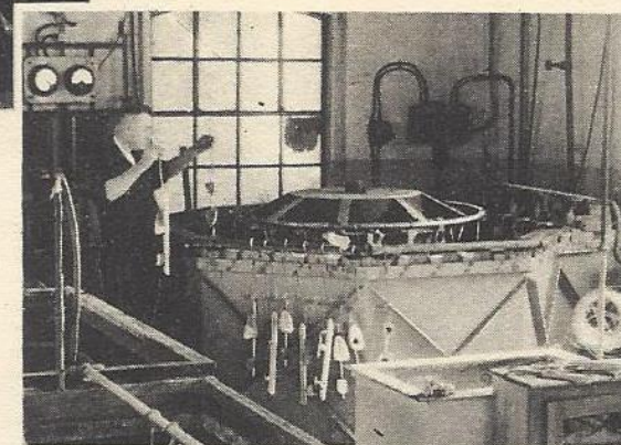
Een kijkje in de galvaniseerinrichting
