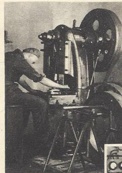
Het uitstampen van onderdelen voor Noorse schaatsen
